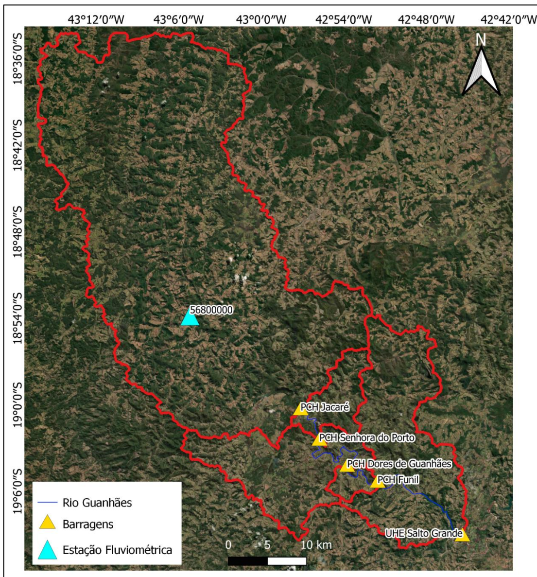
Figura 5-125-13 - Área de contribuição de cada uma das estruturas avaliadas na cascata da PCH Jacaré e da estação fluviométrica utilizada no estudo de vazões máximas
