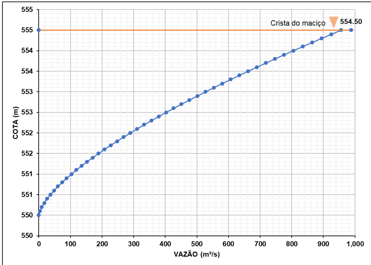
Figura 5-7 – Curva de descarga do vertedouro da PCH Jacaré
