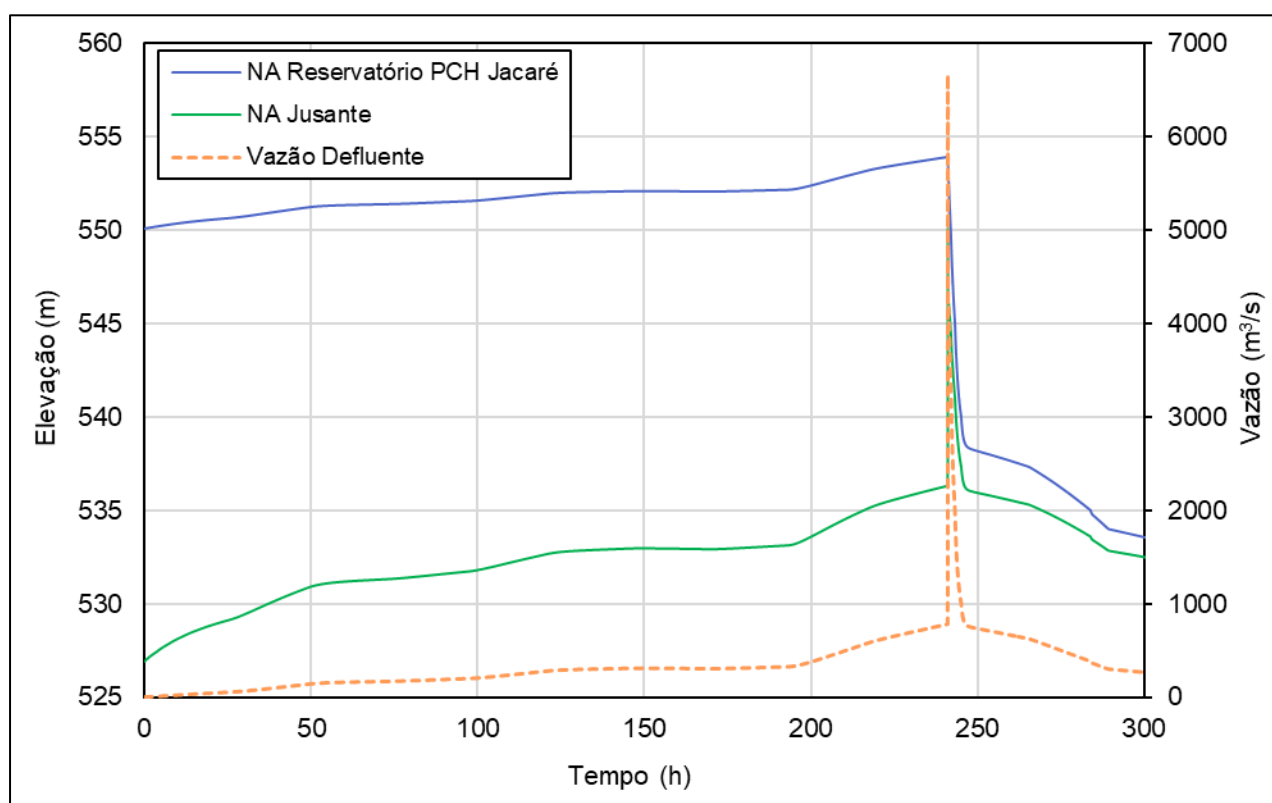
Figura 13-1 – Hidrograma de Ruptura Defluente à PCH Jacaré.
