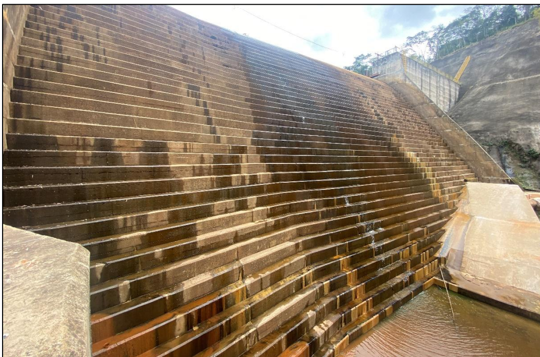
Figura 5-6 – Vista a jusante dos vãos do vertedor da barragem da PCH Jacaré
