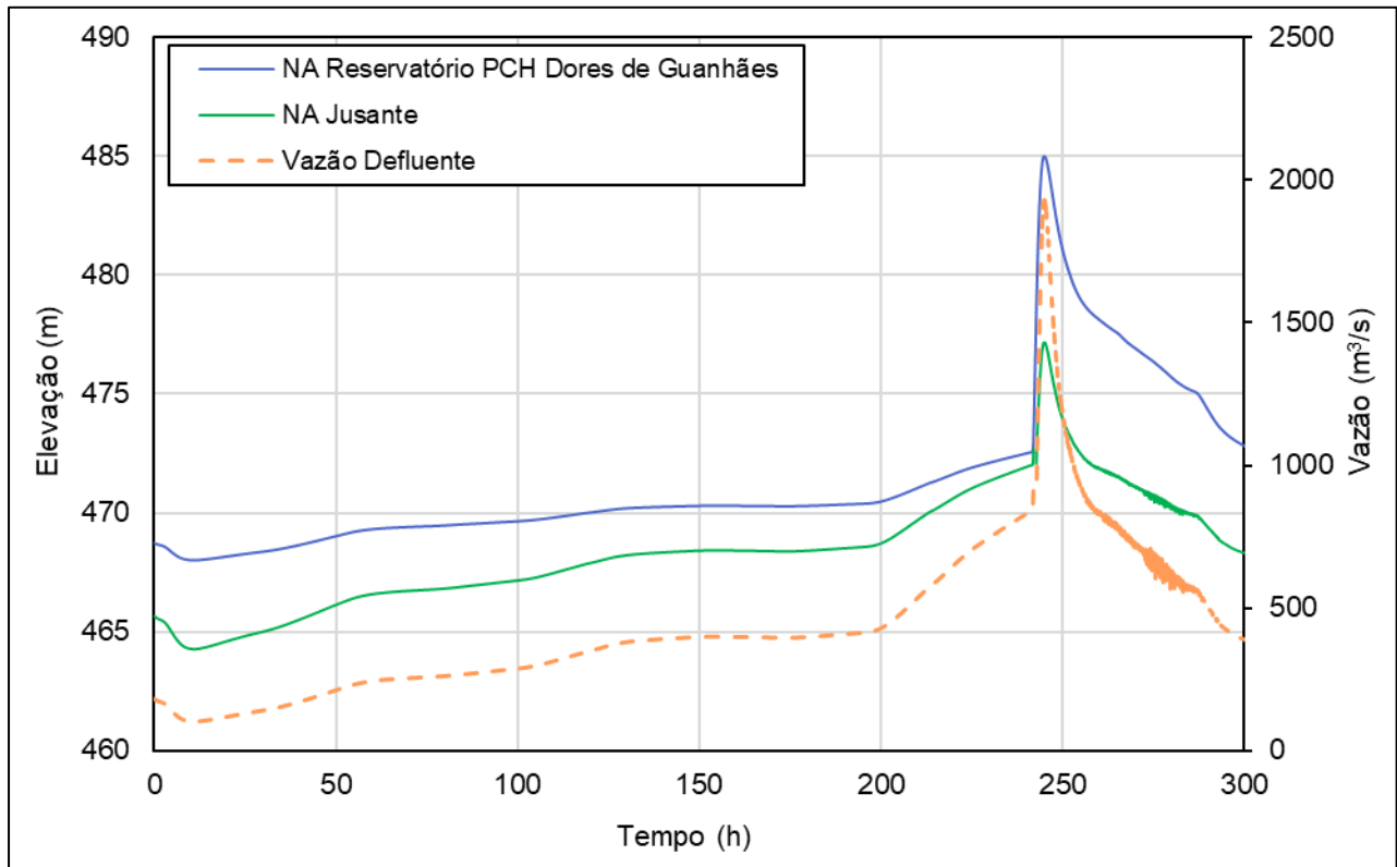
Figura 13-3 – Hidrograma de Ruptura Defluente à PCH Dores de Guanhões.
