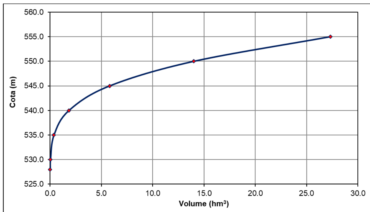
Figura 5-5 – Cota-Volume da PCH Jacaré
