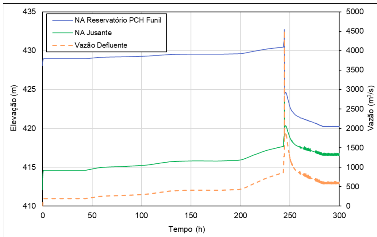
Figura 13-4 – Hidrograma de Ruptura Defluente à PCH Funil.
