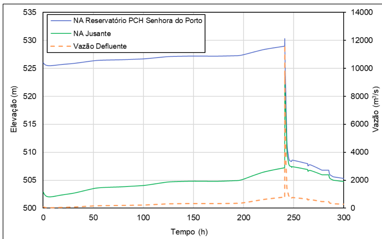
Figura 13-2 – Hidrograma de Ruptura Defluente à PCH Senhora do Porto.
